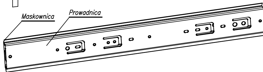
Widok prowadnicy z maskownicą
